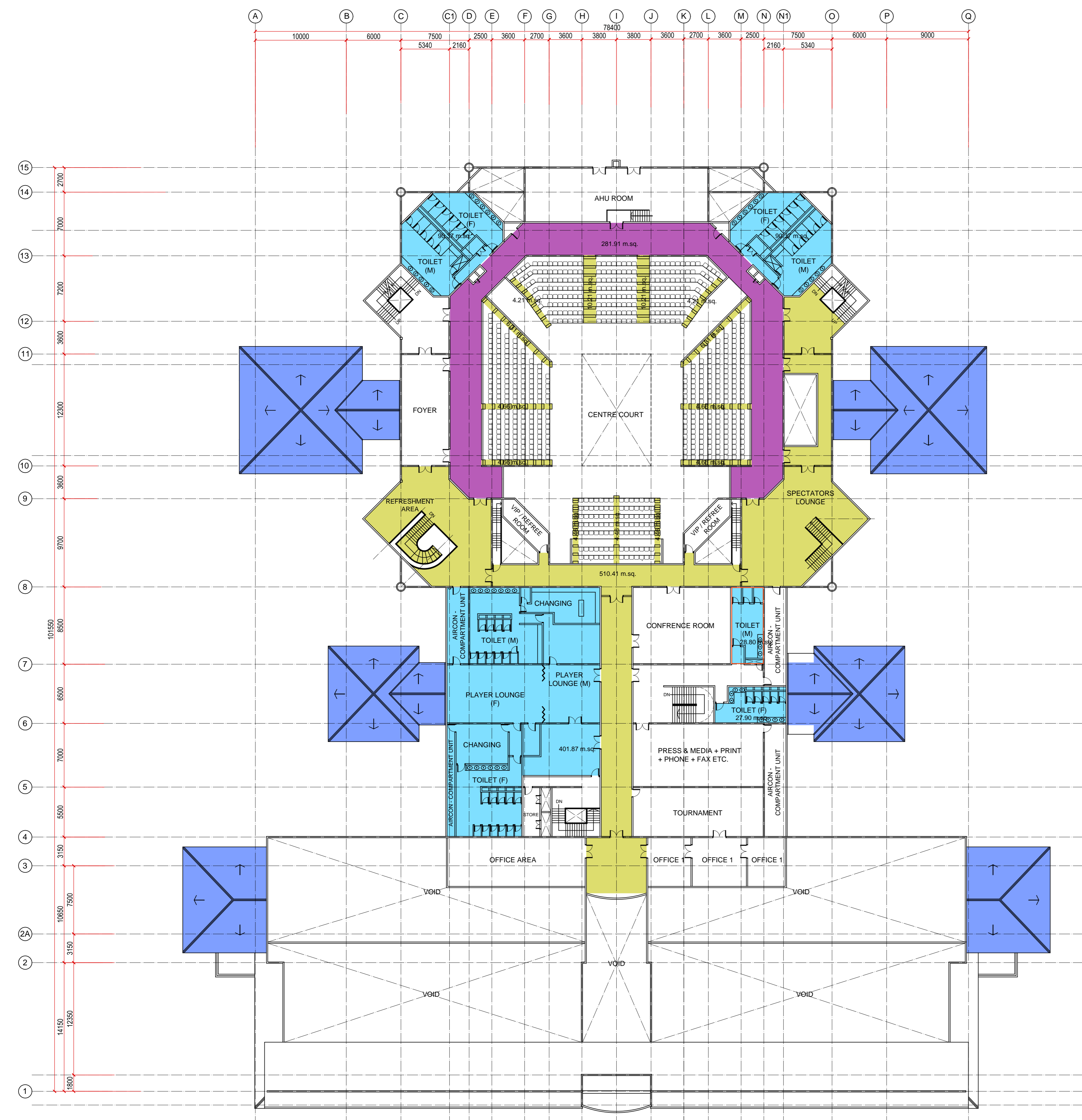
PELAN TINGKAT 1 SKALA 1 : 250
